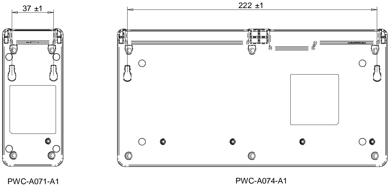
Figura 17-8 Parte inferior do carregador de bateria
