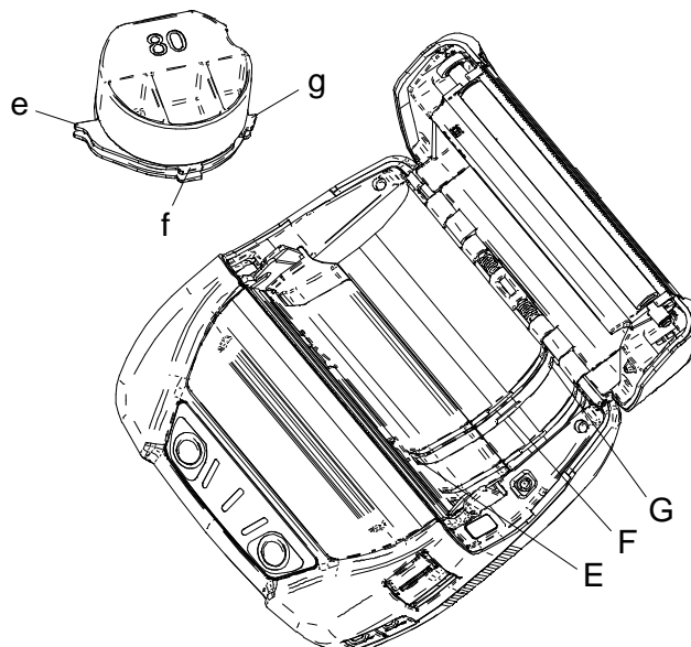
Figura 13-4 Instalação da divisória (1)
