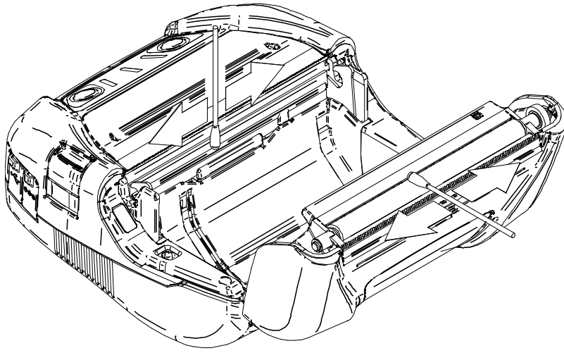
Şekil 18-1 Termal Başlığın/Baskı Levhasının Temizlenmesi
