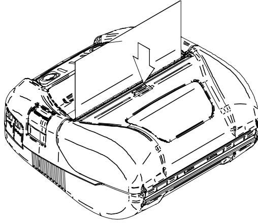
Şekil 9-4 Kağıt Kapağı
