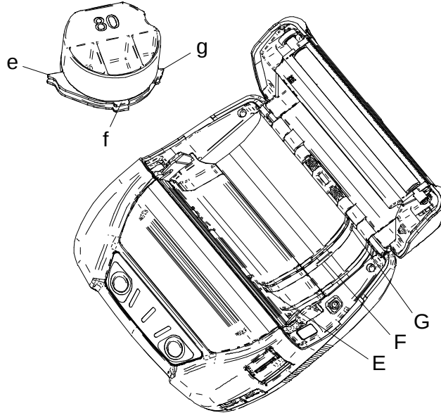
Şekil 13-4 Ayırma Levhasının Takılması (1)
