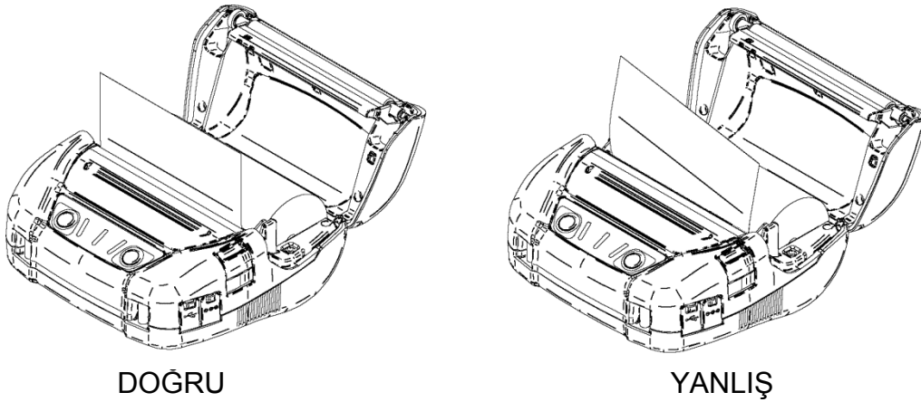
Şekil 9-3 Termal Kağıt Ayarı Yönü Örneği
