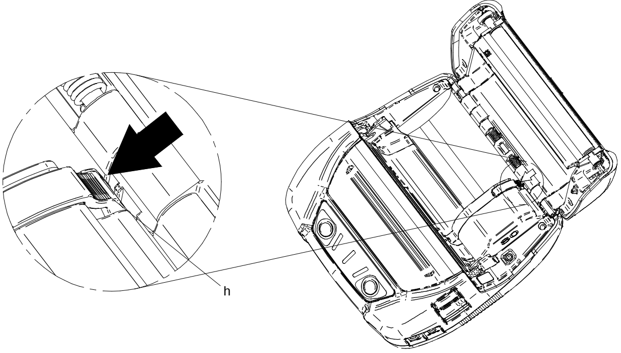
Şekil 13-7 Ayırma Levhasının Çıkarılması
