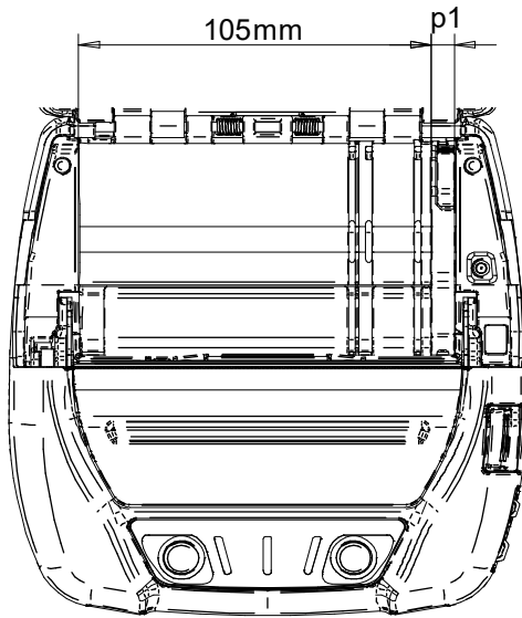
Şekil 13-2 Ayırma Plakası ve Ek Konumu
