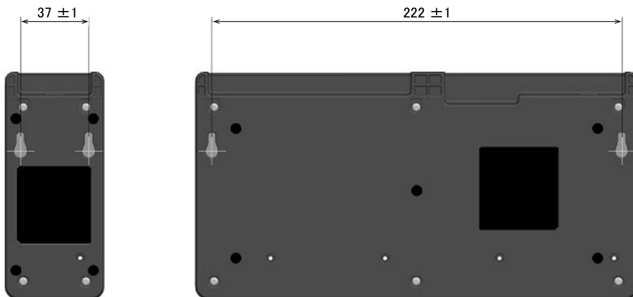
図 17-8 充電器底面図
