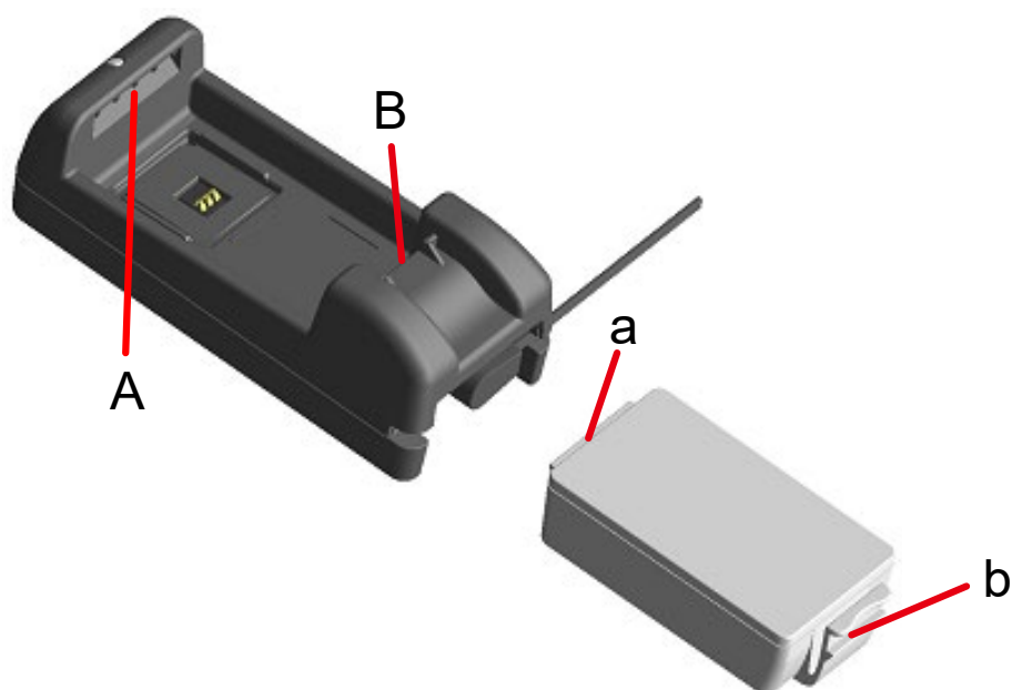
図 17-4 バッテリーパックの向き
