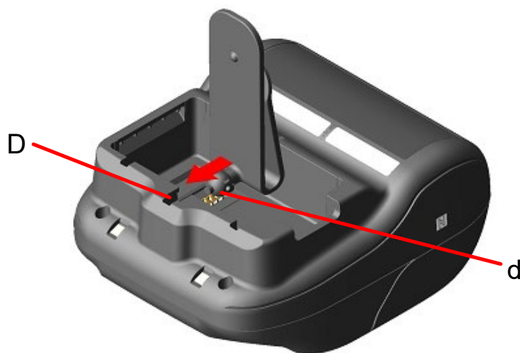
図 13-1 ベルトクリップの取り付け(1)
