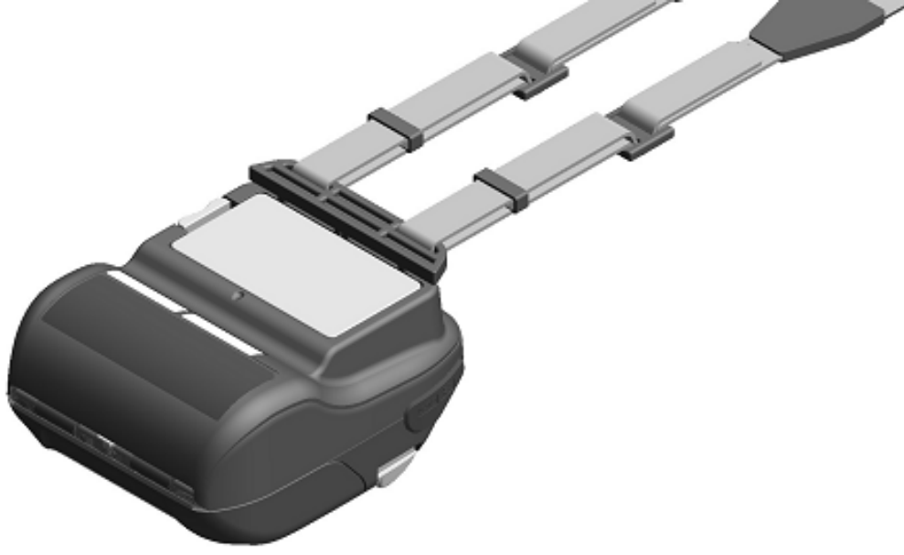
Şekil 13-9 Omuz Kayışının Takılması (5)
