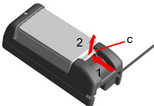
図 18-7 バッテリーパックの充電器からの取り外し
