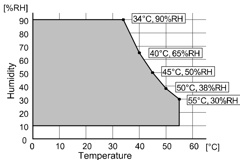
図 21-1 動作温湿度範囲 (印字時)
