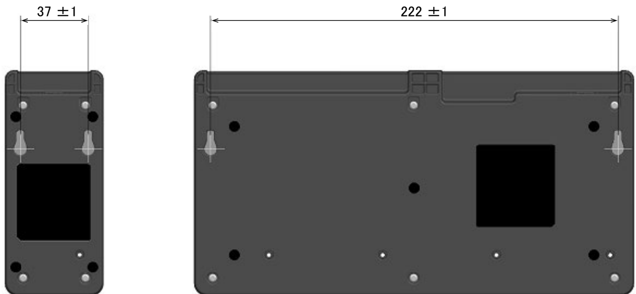
図 18-8 充電器底面図
