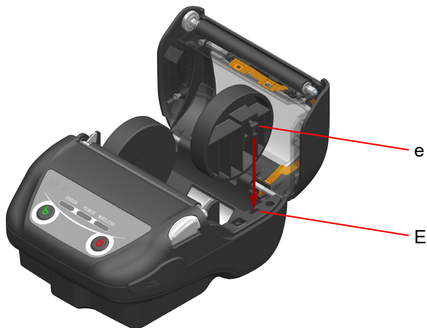
図 14-2 パーテションプレートの取り付け(2)
