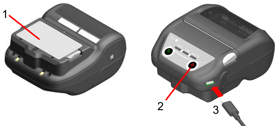
図 16-1 USB ACアダプタによるパワーオン充電モードでの充電
